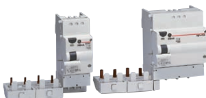
Diff-o-Click FI-Schutzschalter zum Anbau an Leitungsschutzschalter
